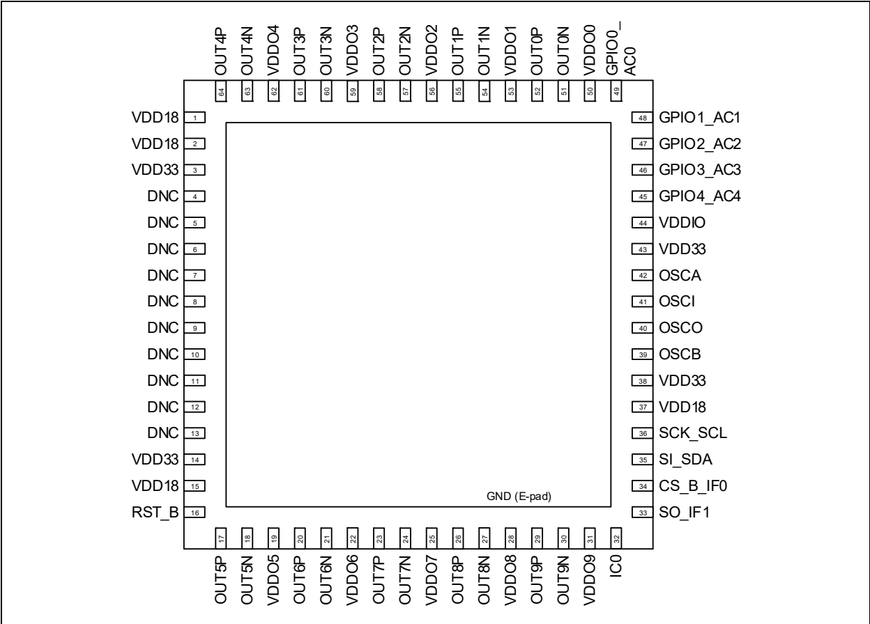
図 3-1: ZL30271 向け 64 ピン 9 mm x 9 mm VQFN (0.5 mm ピッチ )
