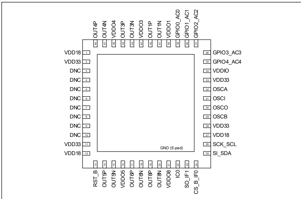
図 3-2: ZL30270 向け 48 ピン 7 mm x 7 mm VQFN (0.5 mm ピッチ)
